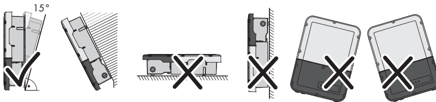
Imagen 5 : Posiciones de montaje permitidas y no permitidas
