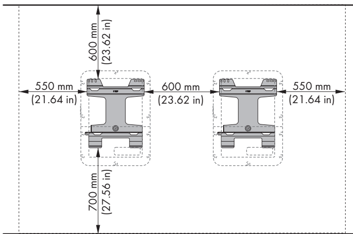
Figure 4 : Distances recommandées (Dimensions en mm (in))
