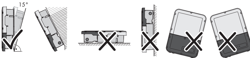
Figure 5 : Positions de montage autorisées et non autorisées
