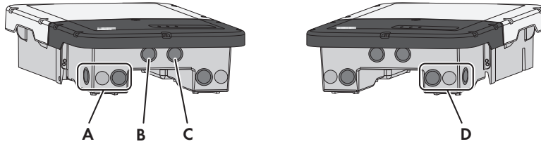
Figure 7 : Ouvertures du boîtier situées sur le dessous de l'onduleur
