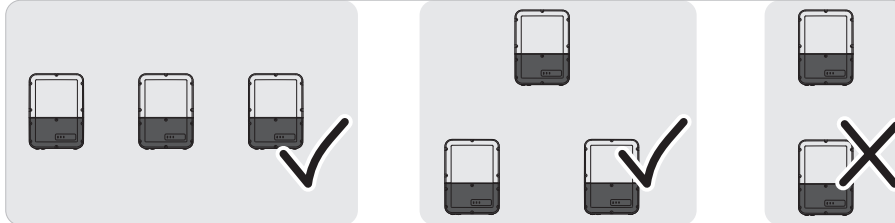
Figure 6 : Positions de montage autorisées et non autorisées de plusieurs onduleurs
