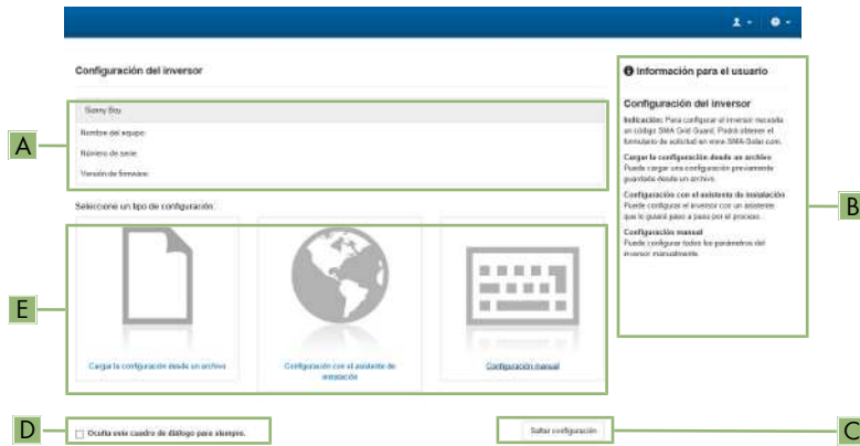
Imagen 10 : Estructura de la página Configurar inversor
