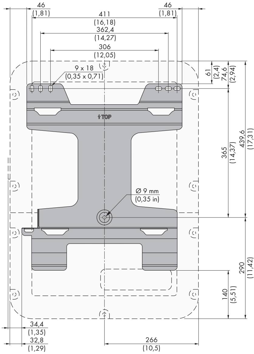
Figure 3 : Position des points de fixation (Dimensions en mm (in))
