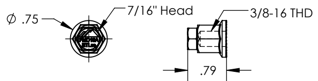
3) NUT, FLANGE, L-FOOT
