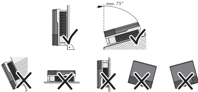
Figure 4 : Positions de montage autorisées et non autorisées
