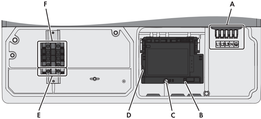
Imagen 6 : Áreas de conexión del interior del inversor
