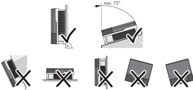
Imagen 4 : Posiciones de montaje permitidas y no permitidas
