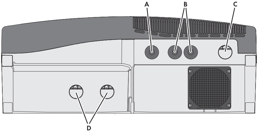
Figure 5 : Ouverture sur le dessous du boîtier de l'onduleur
