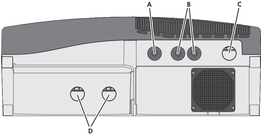
Imagen 5 : Aberturas en la carcasa en la parte inferior del inversor
