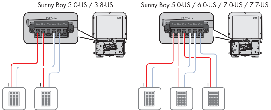
Figure 12 : Vue d'ensemble du raccordement en fonctionnement normal
